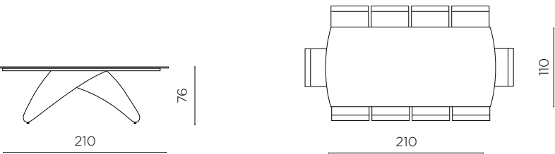
DIMENSIONI / SIZES
